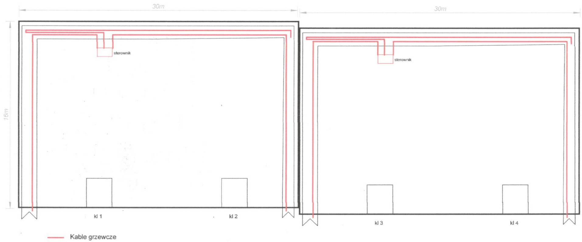
Rzut budynku Widokowe 4
