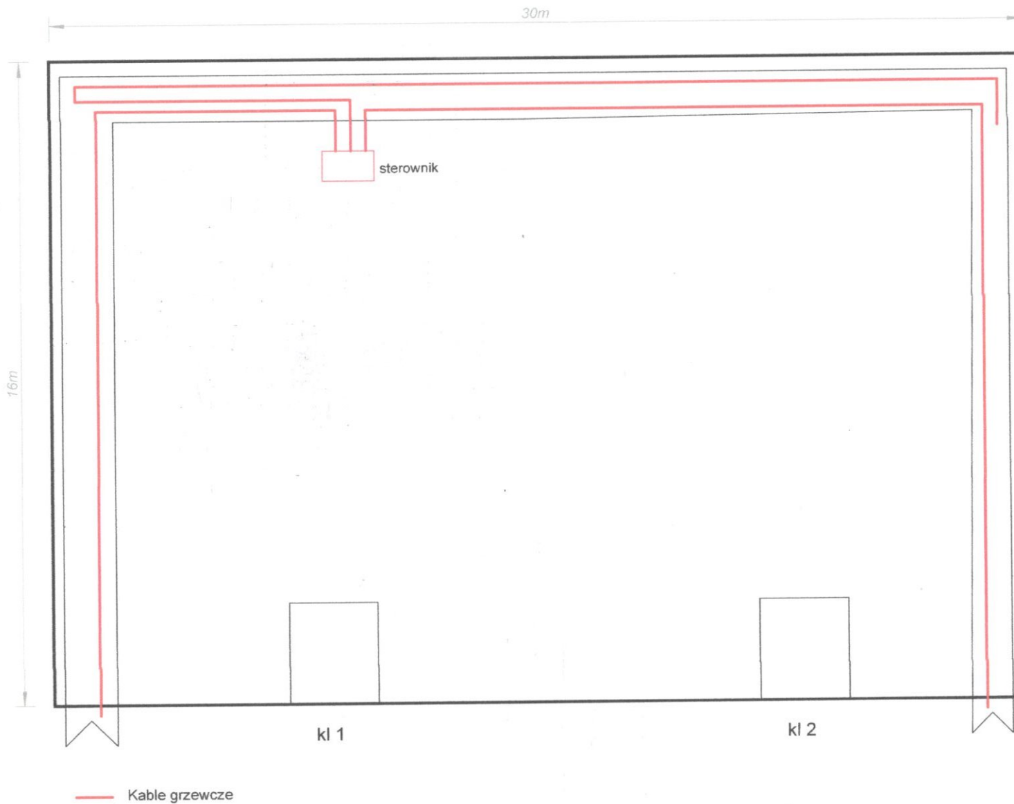
Rzut budynku Kadłubek 30E
