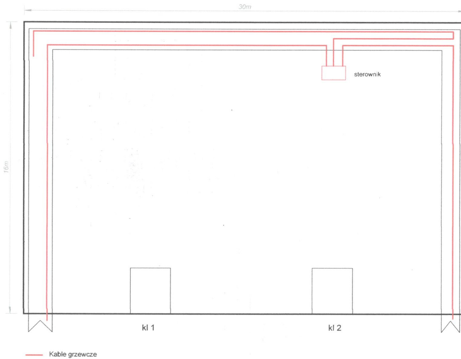
Rzut budynku Kadłubek 30D
