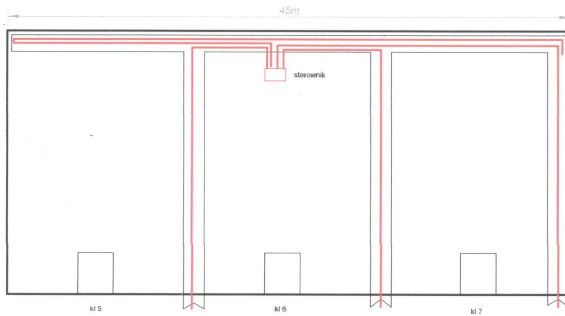
Rzut budynku Wojska Polskiego 5
